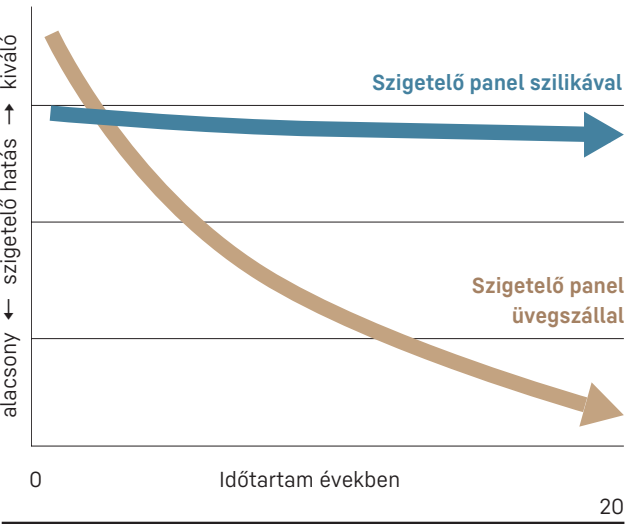
Vákuumszigetelő panelek hatékonysága
